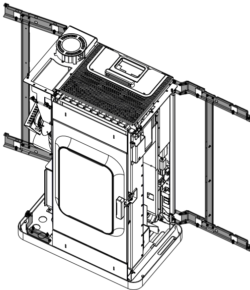
Abb. 19: Tragarme aufklappen
