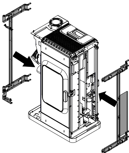
Abb. 17: Tragarme an Pelletofen anbringen
