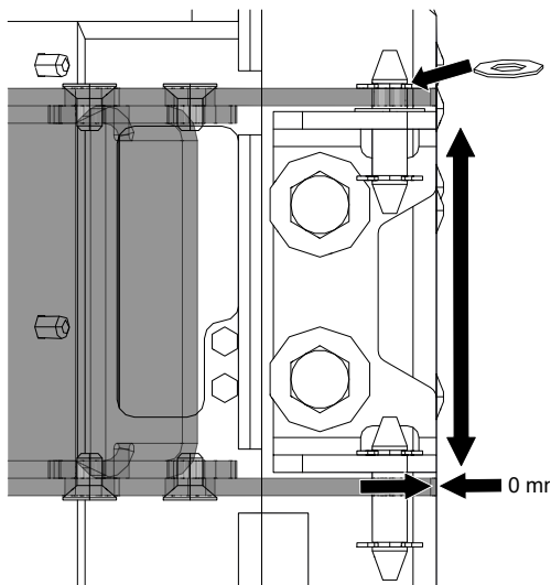
Abb. 20: Höhe der Tragarme einstellen
