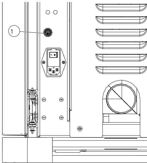
Abb. 97: Sicherheitstemperaturbegrenzer
