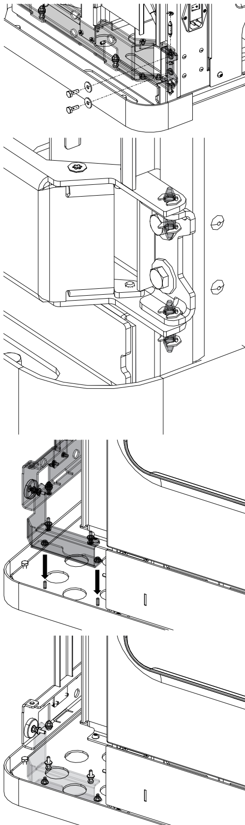
Abb. 18: Tragarme montieren
