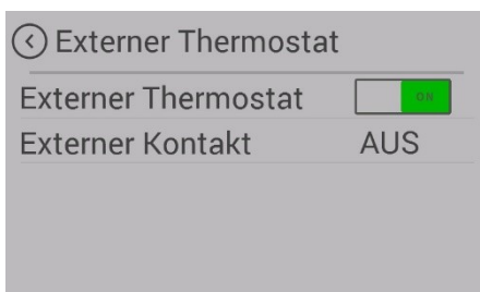
Abb. 67: Externer Thermostat
