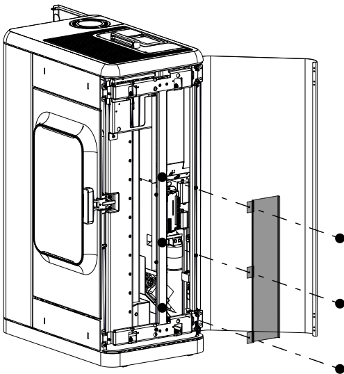
Abb. 34: Abdeckung abmontieren
