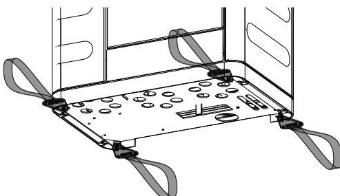
Abb. 6: Transporthilfe
