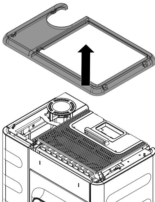
Abb. 10: Deckel abnehmen
