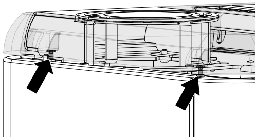
Abb. 31: Deckel einstellen
