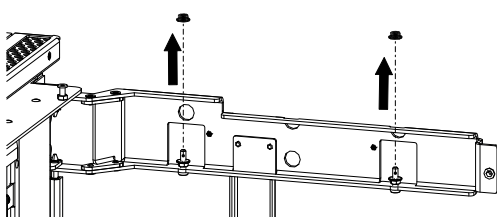
Abb. 21: Muttern lösen
