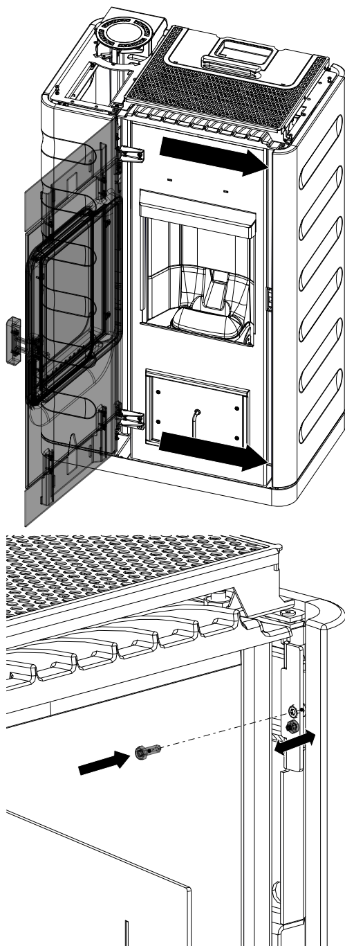
Abb. 23: Keramikverkleidung befestigen
