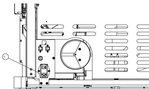
Abb. 47: Elektrischer Anschluss
