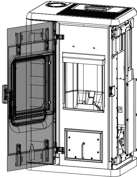
Abb. 99: Tür öffnen
