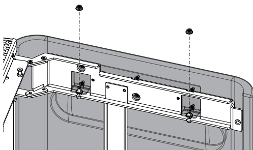
Abb. 22: Keramikverkleidung anbringen
