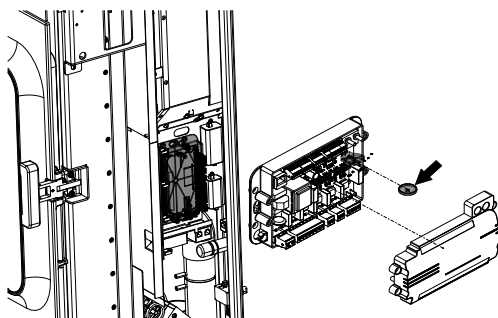
Abb. 83: Speicherbatterie tauschen
