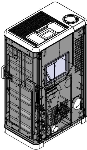
Abb. 44: Rückwand und Seitenverkleidungen montieren
