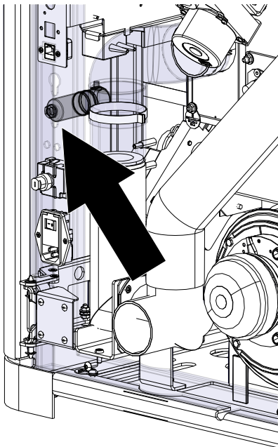
Abb. 37: Kabel durchziehen
