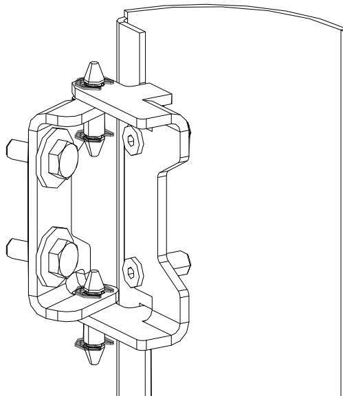
Abb. 27: Stahlverkleidung am Pelletofen montieren
