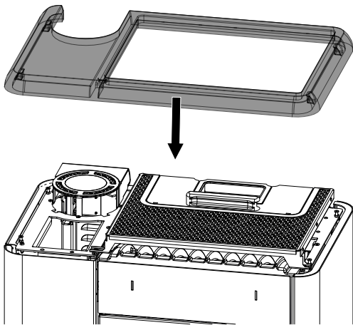
Abb. 30: Deckel anbringen
