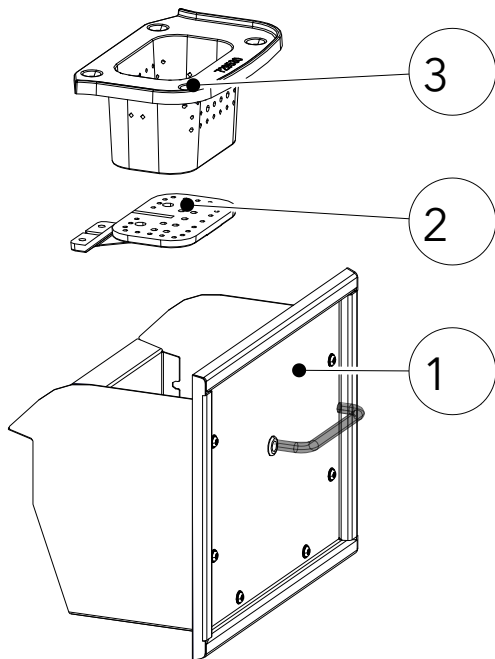
Abb. 84: Kipprost reinigen
